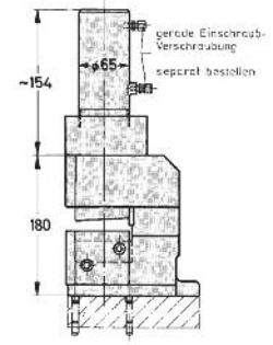
Antrieb hydr. doppelwirkend Serie 660-063-..
