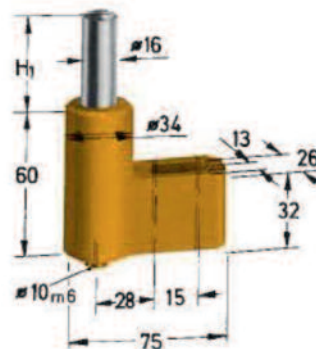
Werkstückanschlag
